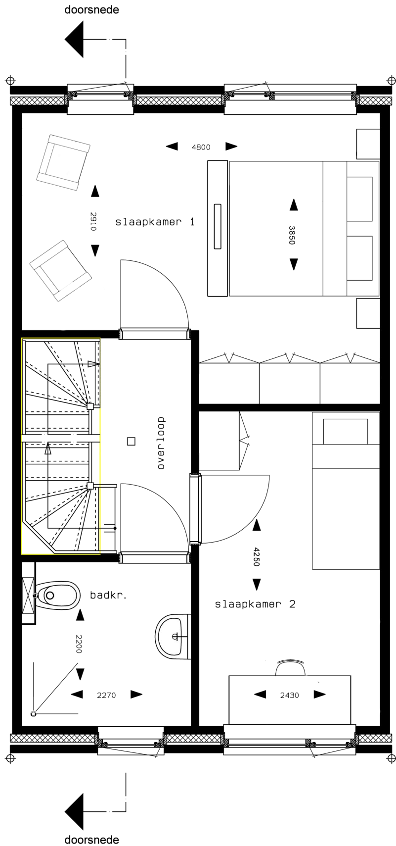
plattegrond verdieping 1:50
